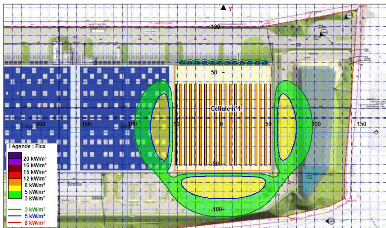
Figure 1 : Flux thermiques associés à l'incendie de la cellule 1
